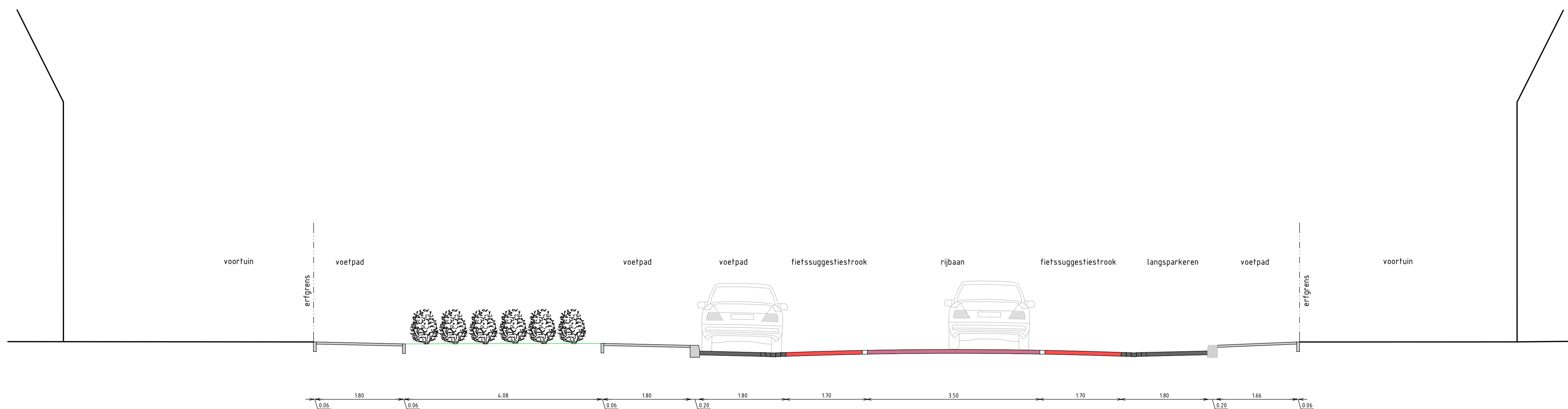
Doorsnede A-A Schaal 1:50
